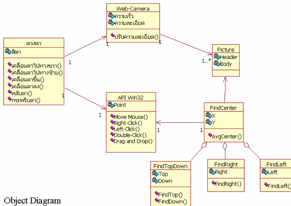
รูปที่ 6-7 Object Diagram ของเมาส์
